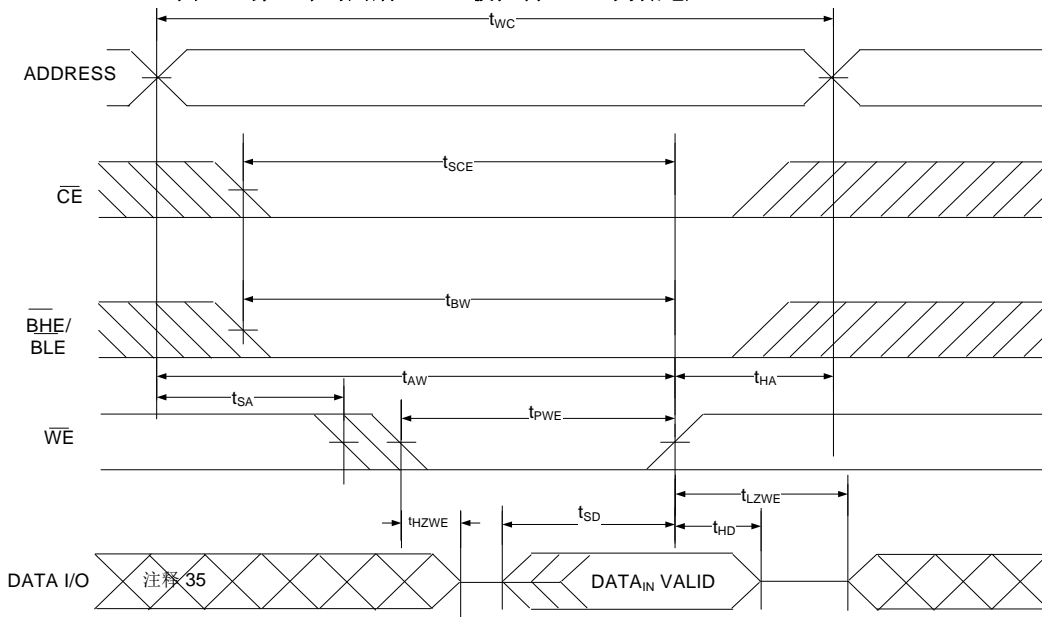
图 17. 第二个写周期 ( \overline{WE} 被控制, \overline{OE} 为低电压) [31、32、33、34]
