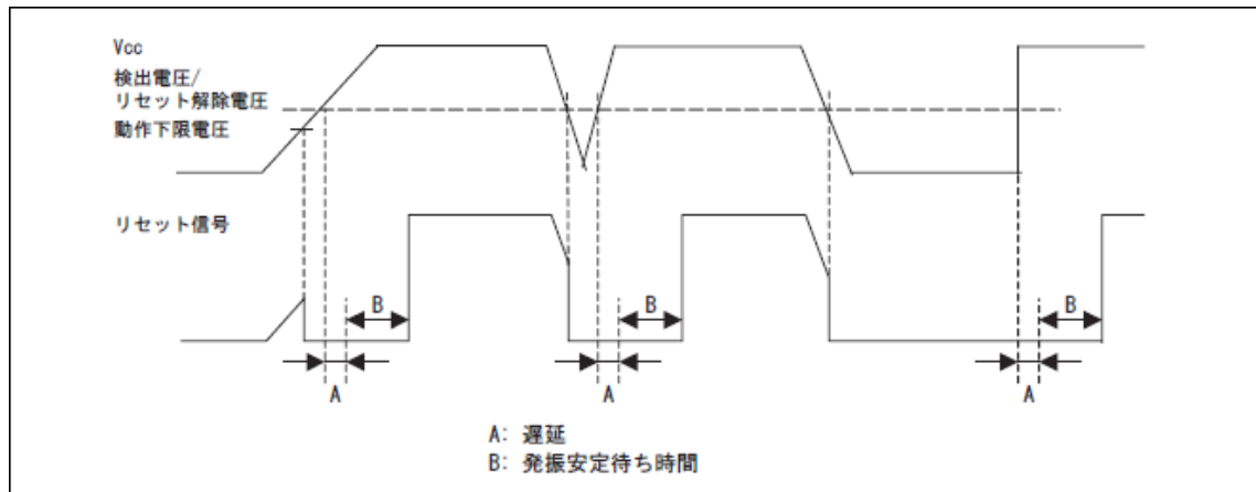
図 3. 低電圧検出リセット回路の動作
