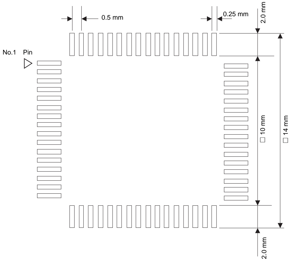
図 4-2. NQPACK 実装用推奨フットパターン寸法図
