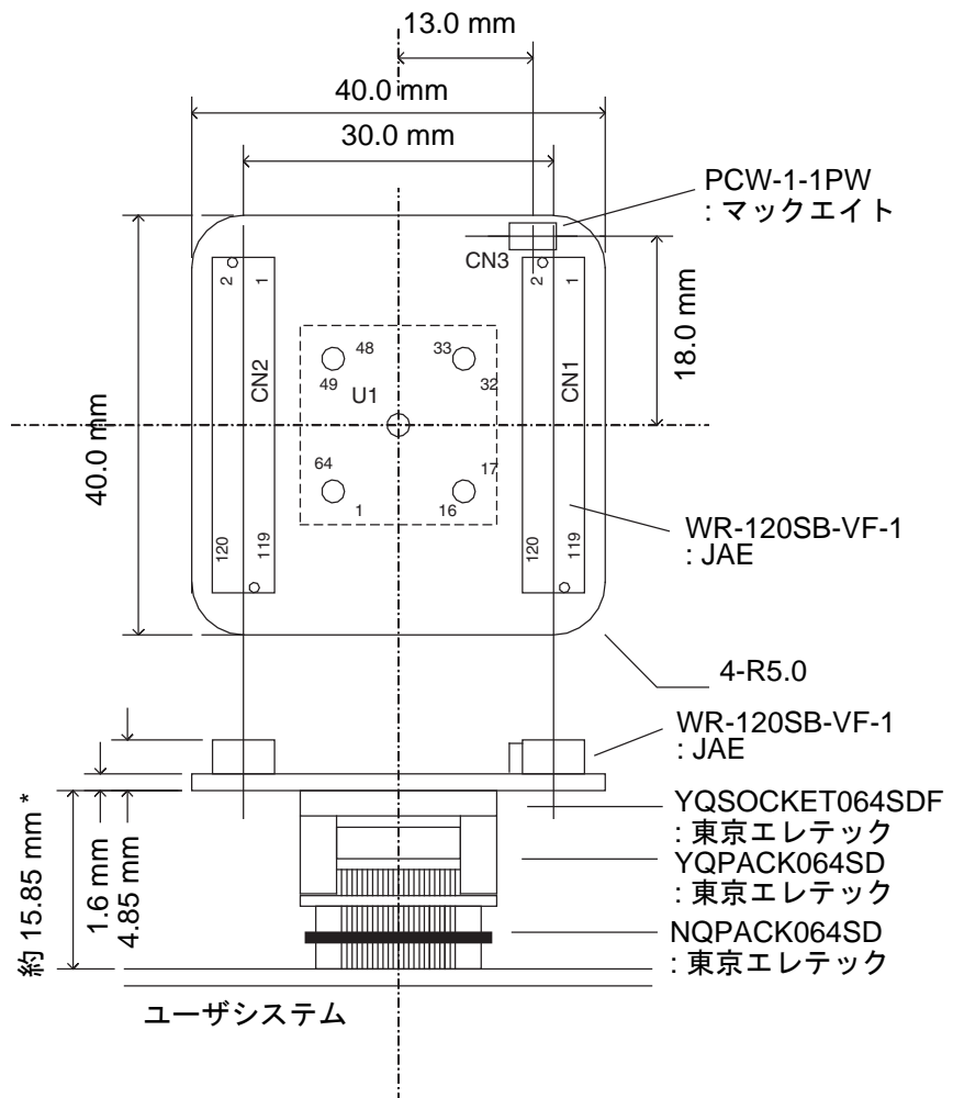
図 4-1. ヘッダボード寸法図
