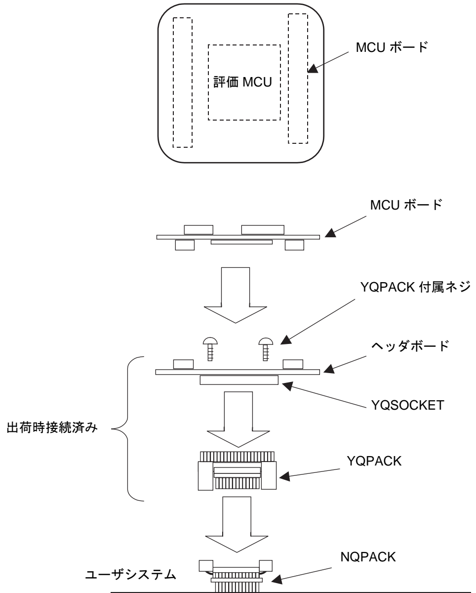
図 5-2. MCU ボード / ヘッダボードのユーザシステムへの接続
