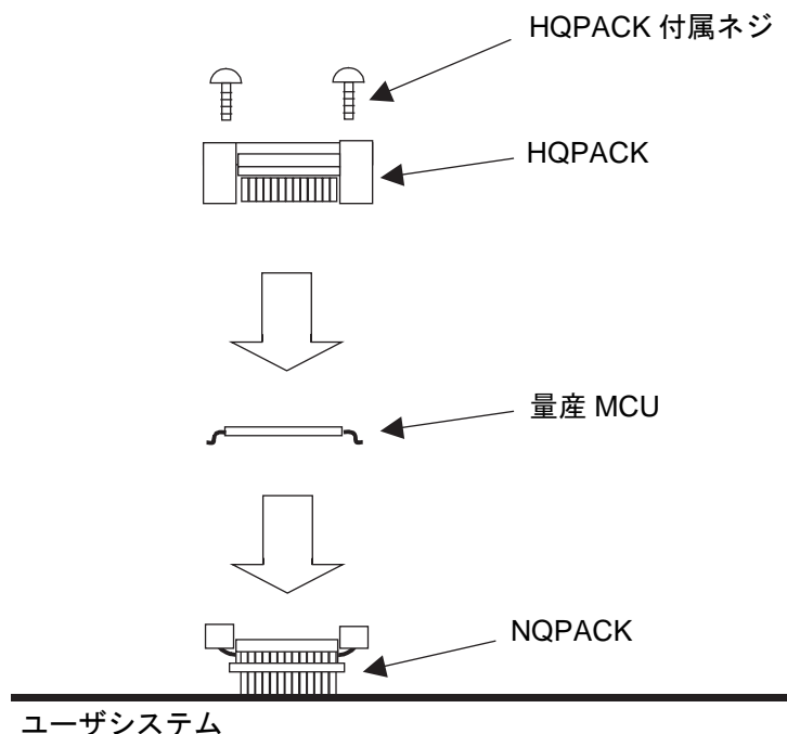
図 6-1. 量産 MCU の実装方法
