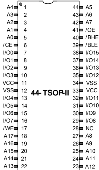
图 3. 44-TSOP II 引脚分布 (单芯片使能), CY62147GN [2]
