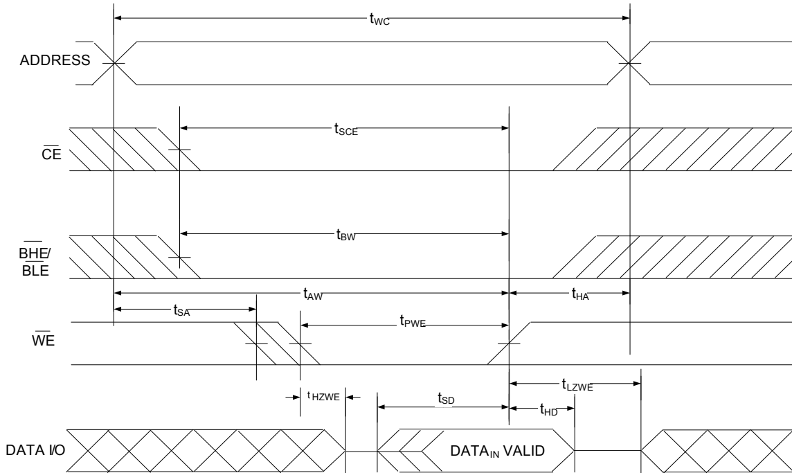
图 9. 第一个写周期 (由 \overline{WE} 控制) [25、26、27]
