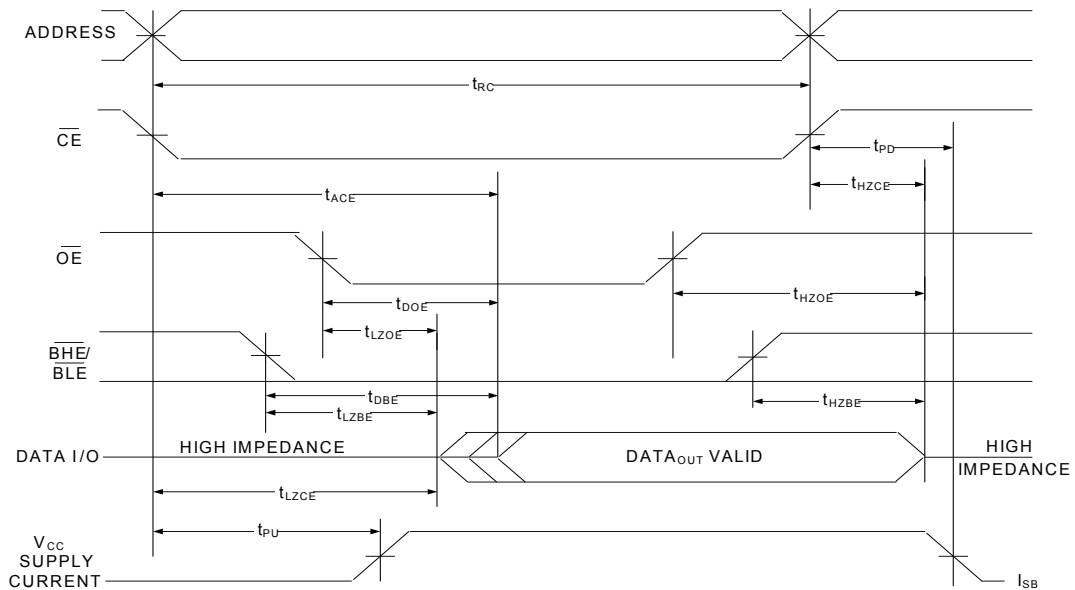
图 8. 第二个读周期（由 \overline{OE} 控制） [21、22、23、24]
