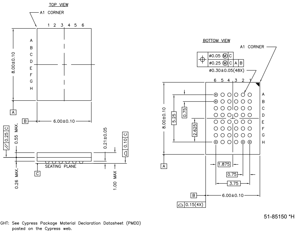
图 14. 48 球 VFBGA (6 × 8 × 1.0 mm) BV48/BZ48 封装外形 — 51-85150
