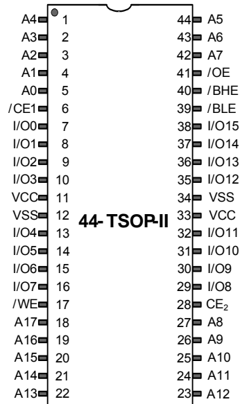
图 4. 44-TSOP II 引脚分布 (双芯片使能), CY621472GN
