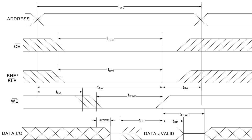
图 11. 第三个写周期 (由 \overline{WE} 控制, \overline{OE} 为低电平) [28、29、30、31]
