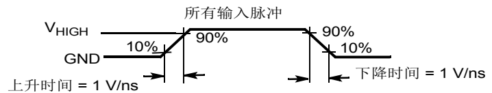
图 5. 交流测试负载和波形 [8]
