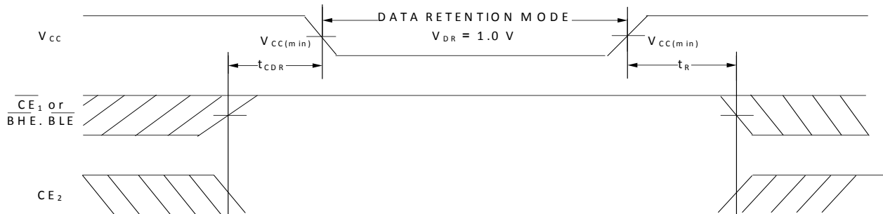
图 6. 数据保持波形 [14]
