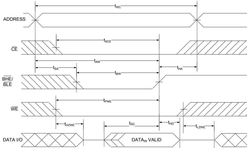
图 12. 第四个写周期 (由 \overline{\text{BHE}}/\overline{\text{BLE}} 控制) [32、33、34]
