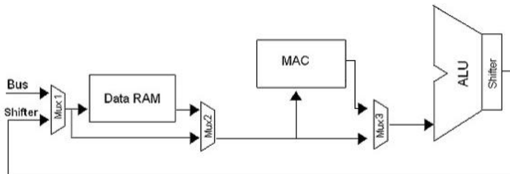
图 4. 数据路径
