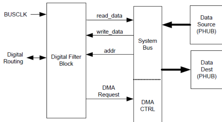
图 2. DFB 应用图
