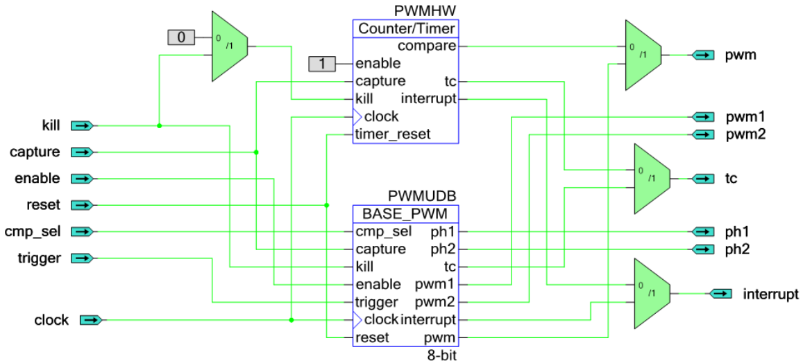
图 4. 顶层原理图
