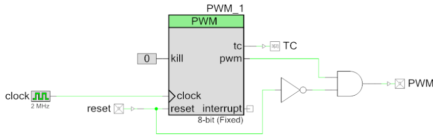
图 3. 固定功能 PWM 实现原理图
