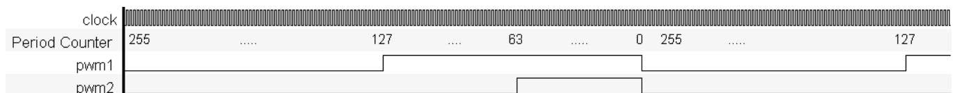
图 1. PWM 输入和输出
