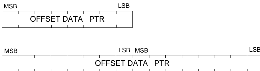
图 2.8 位和 16 位辅助地址大小（自上而下）
