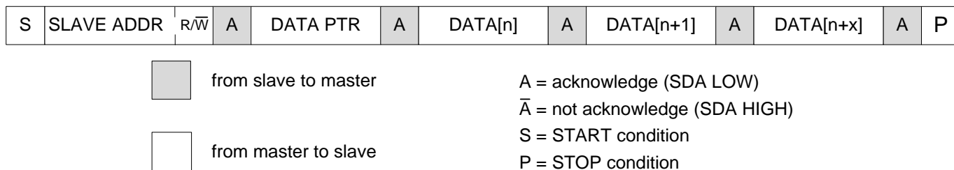
图 3. 将 (x+1) 字节写入 I 2 C 从器件
