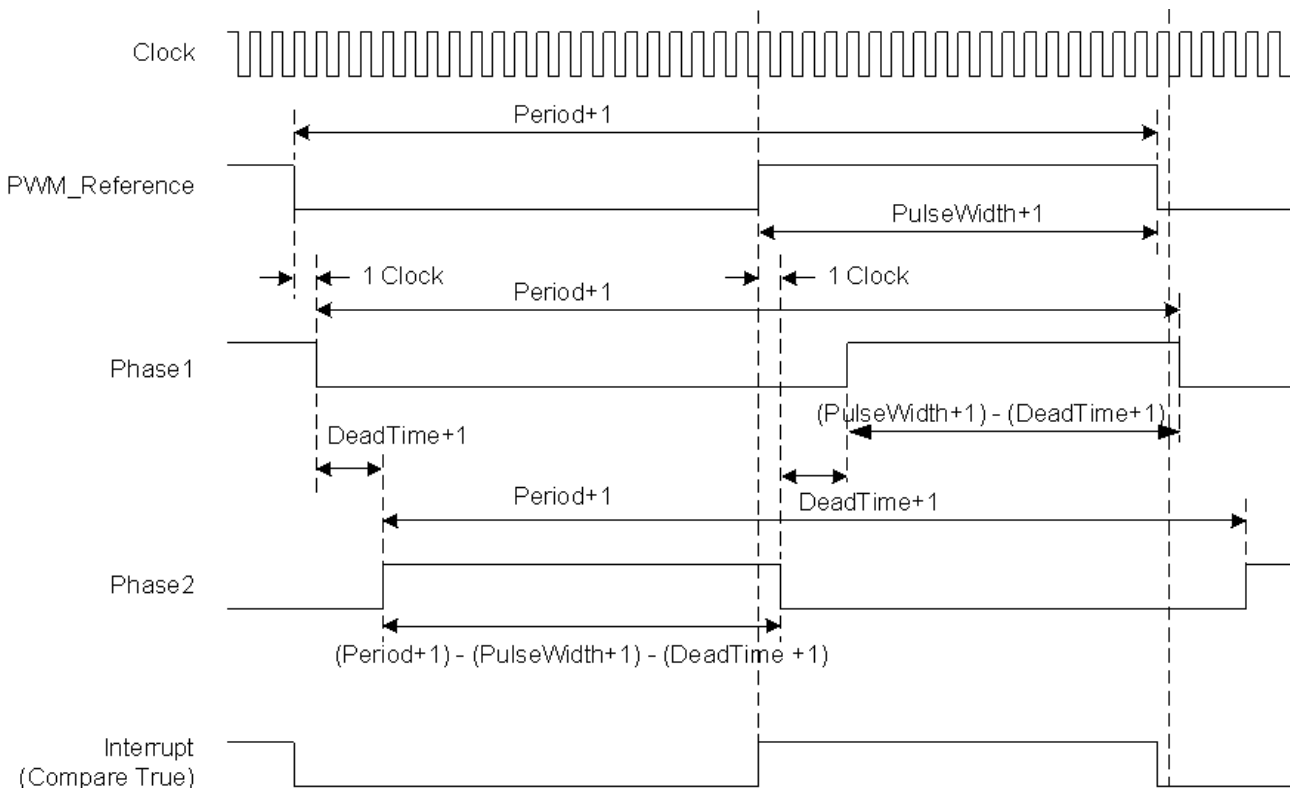
Figure 4. PWMD8L 时序框图
